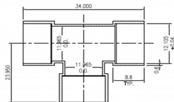
TEE
