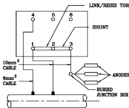
TCP GALVANIC ANODE INSTALLATIO (CONNECTION SCHEME-I)
